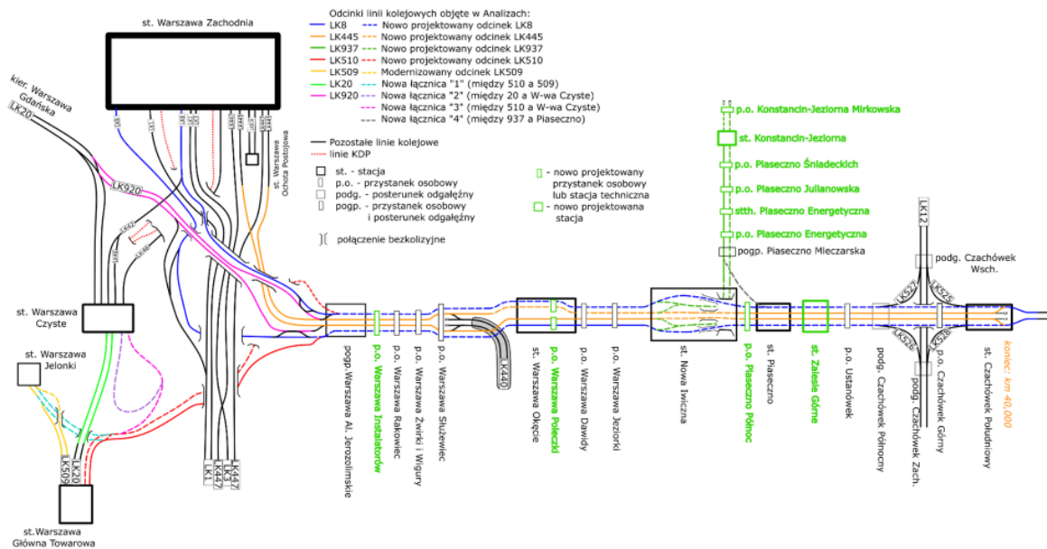
Ryc. 19: Schemat projektu „Dobudowa torów aglomeracyjnych na odcinku Warszawa Al. Jerozolimskie - Piaseczno wraz z połączeniem do Konstancina – Jeziornej”
