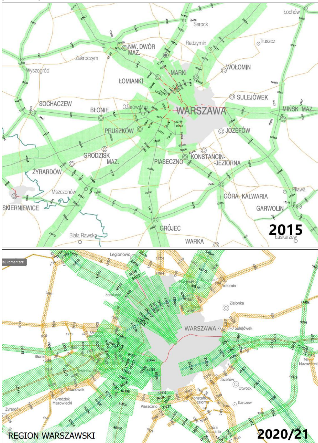
Ryc. 7: Średni dobowy ruch roczny pojazdów silnikowych na podstawie wyniku generalnego pomiaru ruchu (GDDKiA) w latach 2015 i 2020/21
