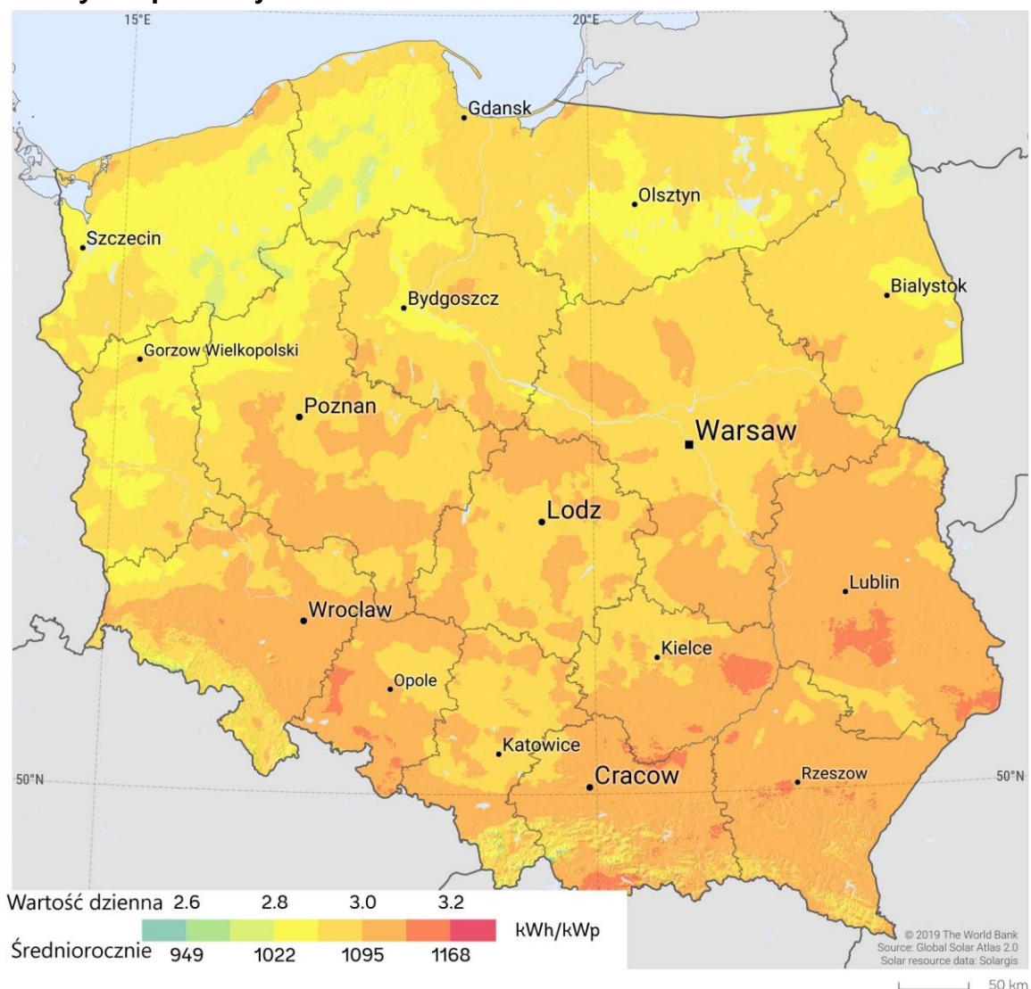
Ryc. 49: Mapa potencjału wydajności instalacji fotowoltaicznej o mocy 1 kWp na płaszczyźnie poziomej na obszarze Polski
