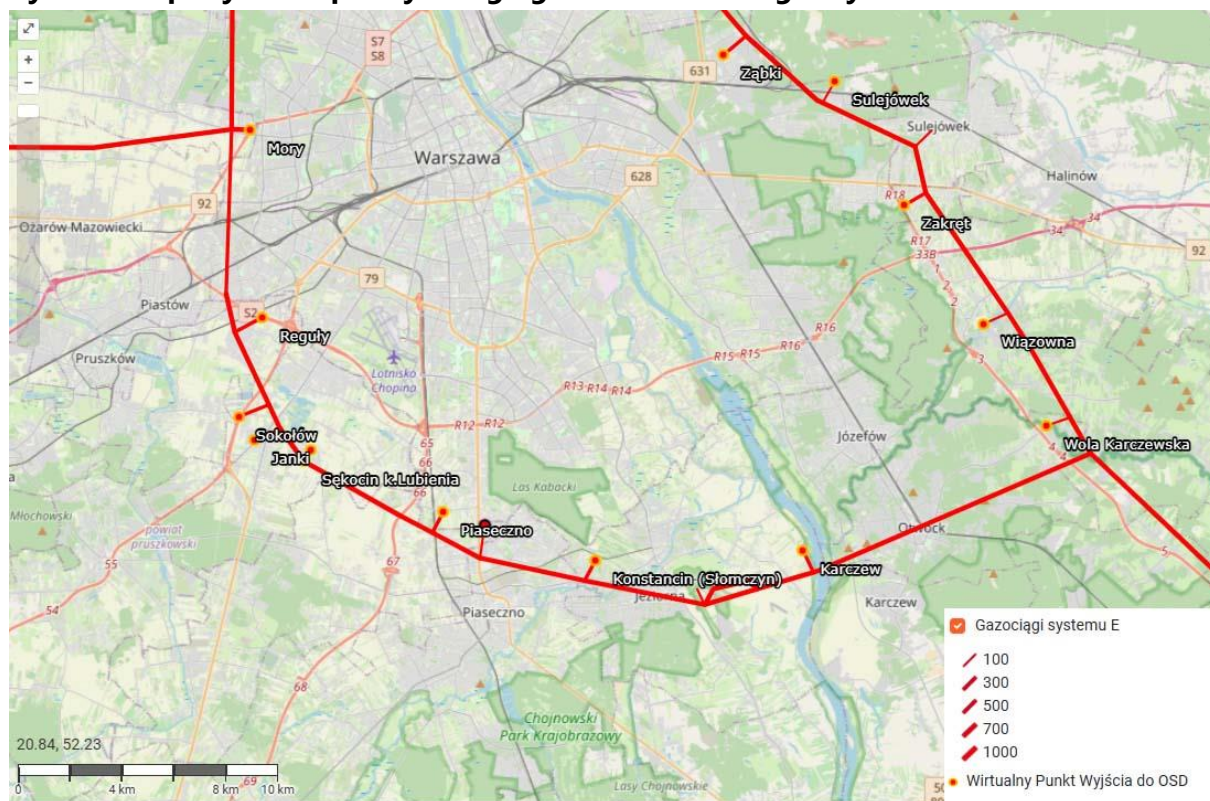
Ryc. 46: Mapa systemu przesyłowego gazu na obszarze gminy Konstancin-Jeziorna
