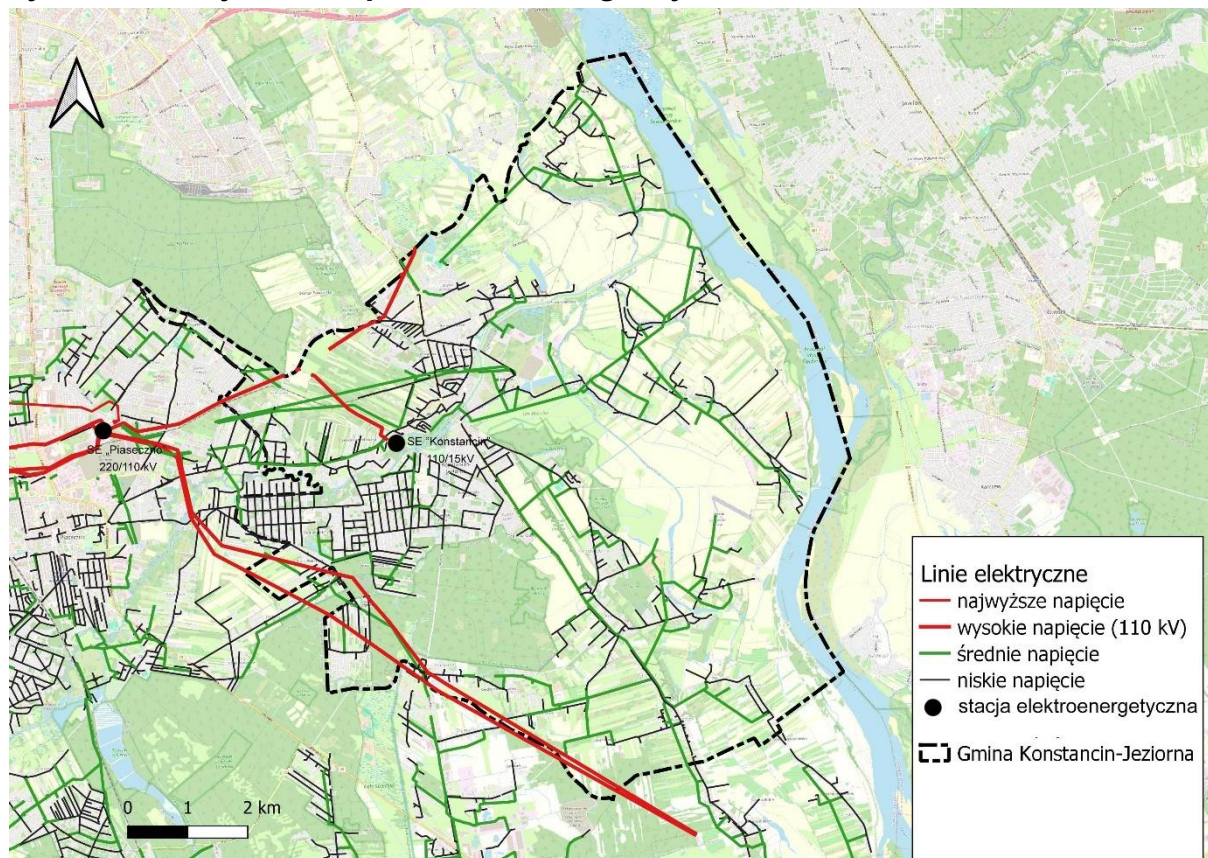
Ryc. 47: Linie wysokich napięć na obszarze gminy Konstancin-Jeziorna
